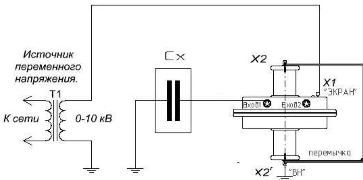
Рисунок 5. «Перевернутая» схема измерений
