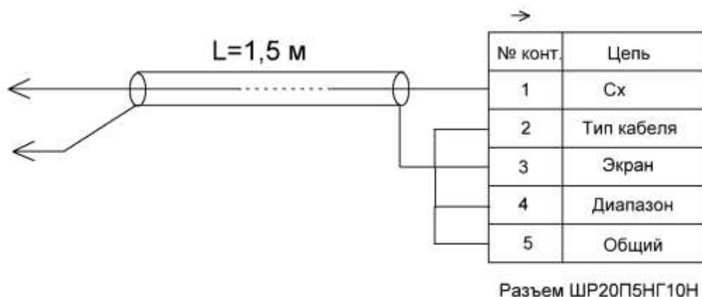
Рисунок 7 а. Схема монтажная кабеля соединительного КС-1.
